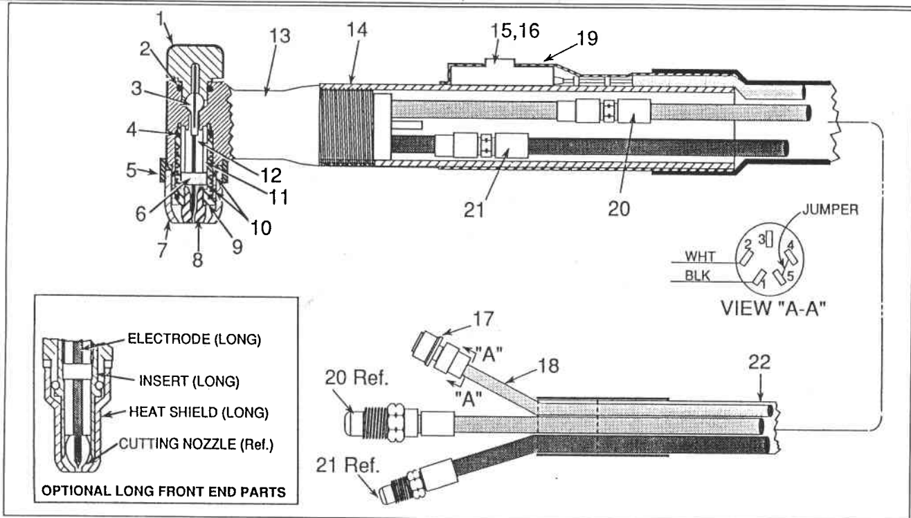
Fig. A PT-150 Torch
